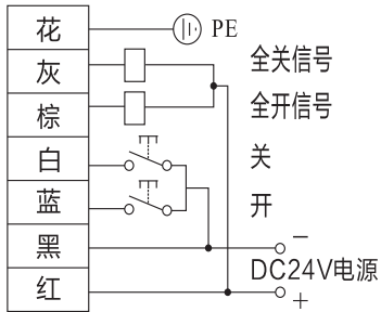
控制电路
