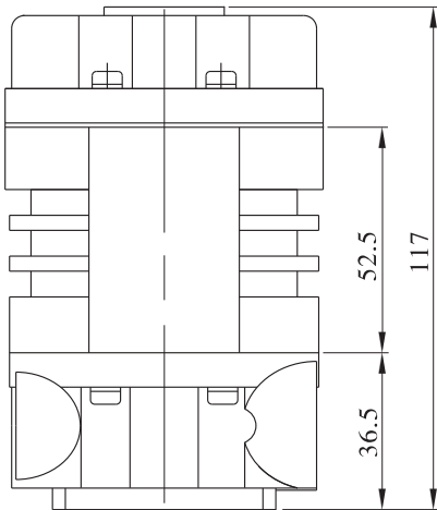
外型尺寸图
